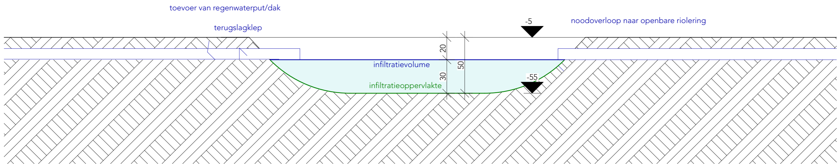
principetekening bovengrondse infiltratie / WADI dwarsnede
