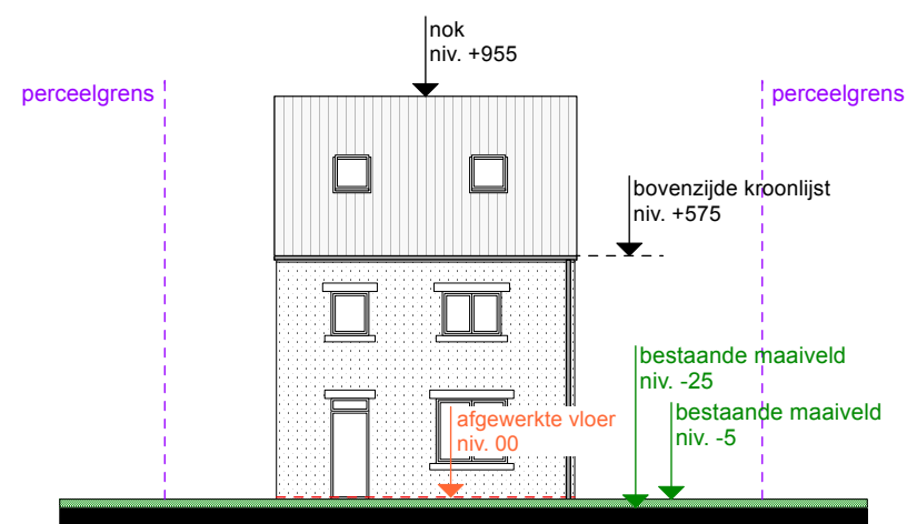
TERREINPROFIEL 2
