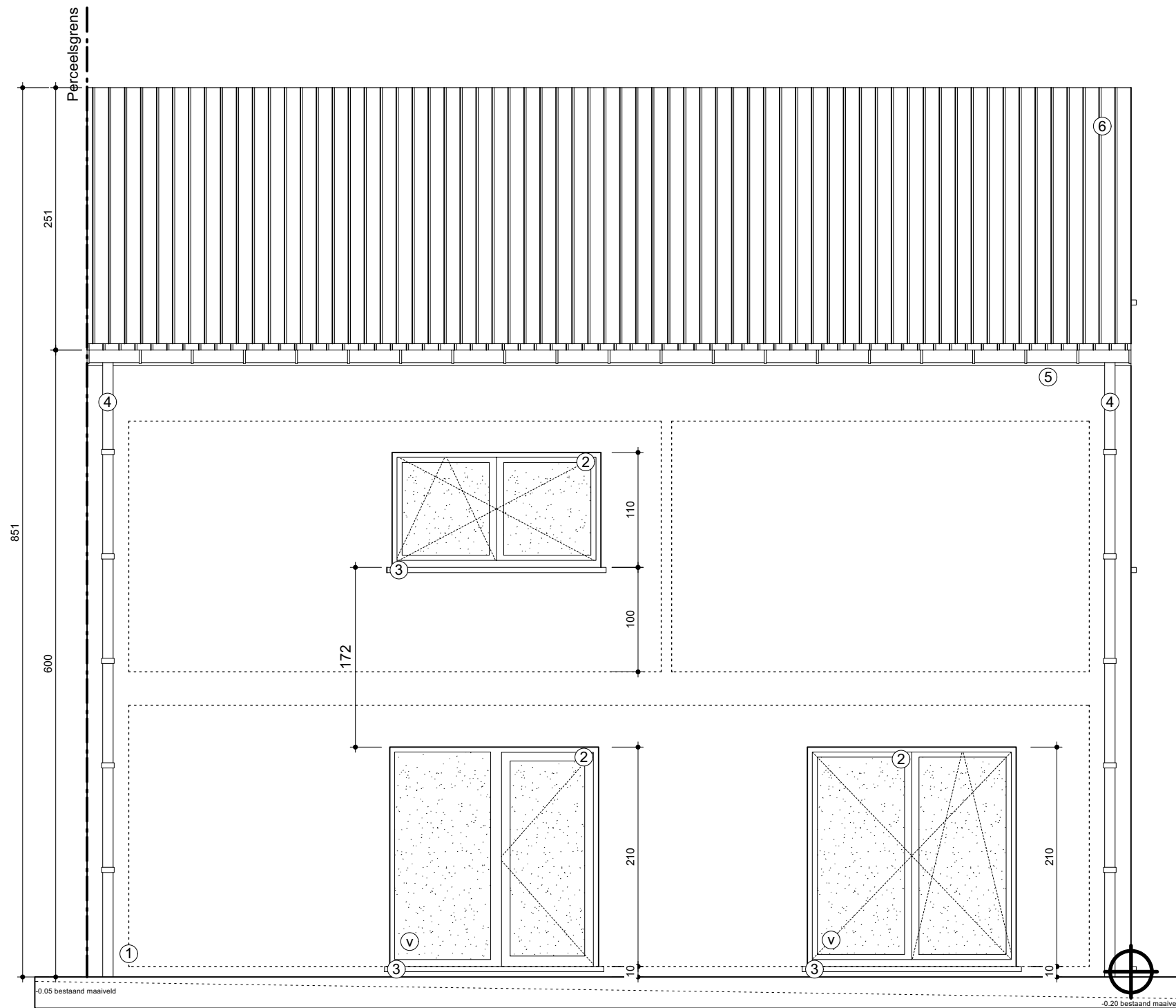
Achtergevel AG Schaal: 1:50
