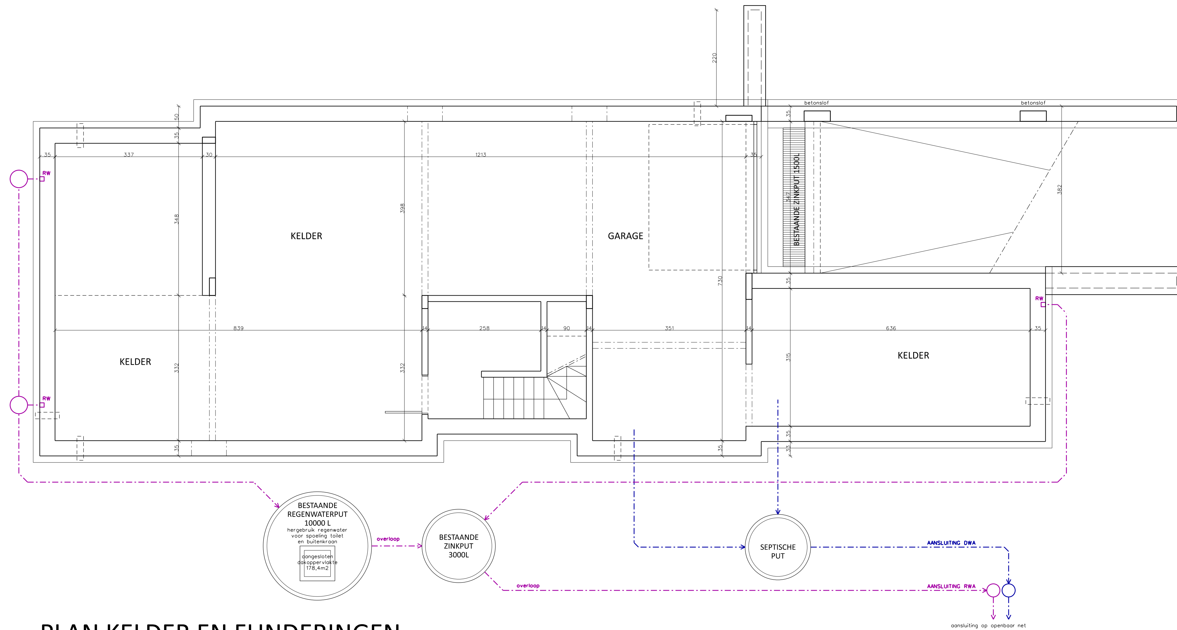
PLAN KELDER EN FUNDERINGEN
